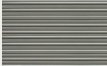
Urano
