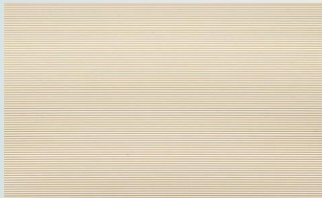
V1006
